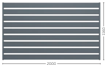
Wersja FORTE 100 9 paneli w przęśle
